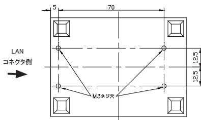
底面のネジ穴（全モデル共通）
