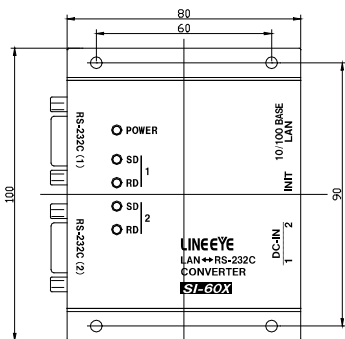
別売りの L 型金具 (SI-ML1) 装着状態
