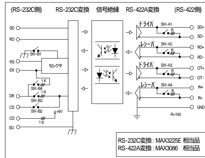
本機内部の信号変換回路ブロック図
